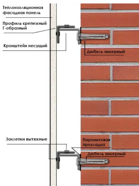
Рис.1. Конструкция НФС «АЛПАН»
