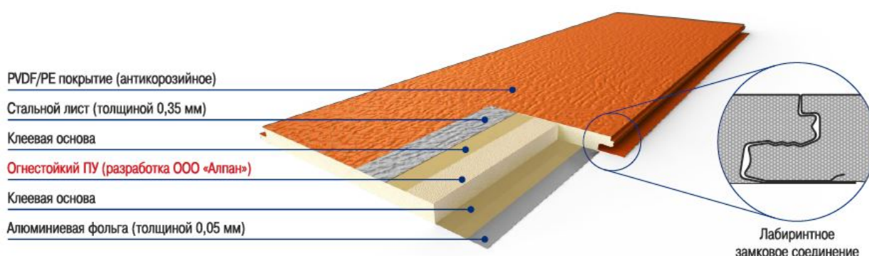
Рис.2. Трёхслойная фасадная теплоизоляционная панель «АЛПАН».
