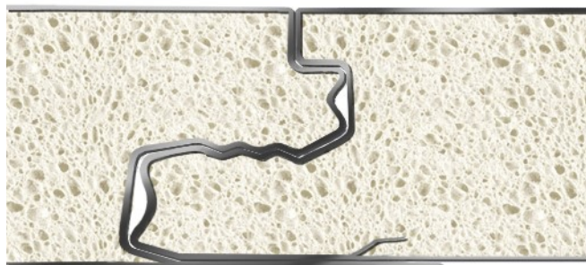
Рис.4. Лабиринтное замковое соединение
