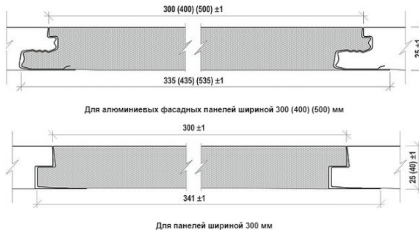
Рис.3. Основные параметры алюминиевых панелей
